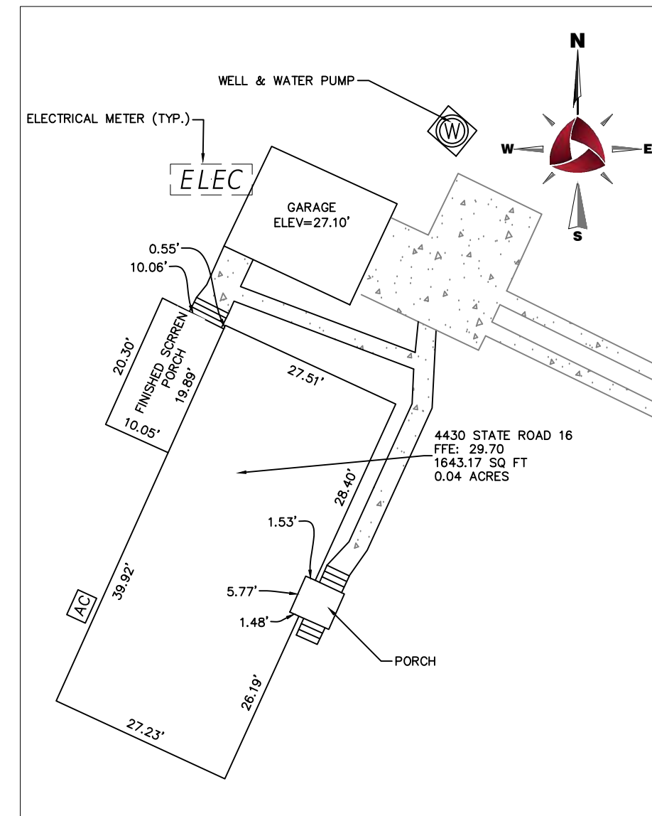
DETAIL "B" SCALE: 1" = 20'
